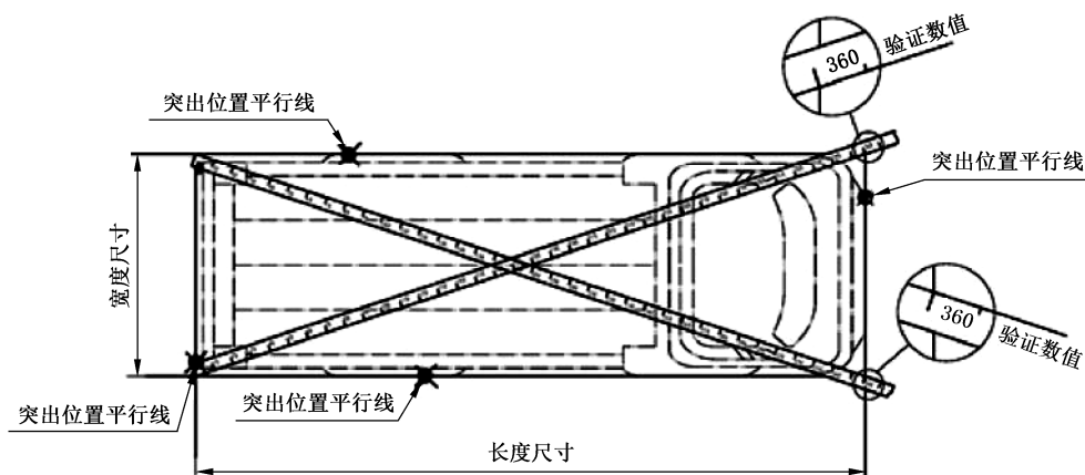
图 B.2 车辆长度、宽度的测量示意
