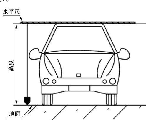
图 B.3 车辆高度的测量示意
