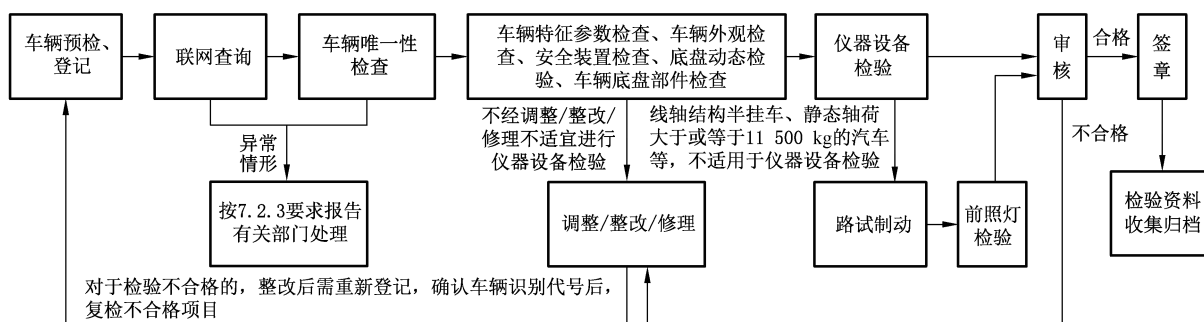
图 A.1 机动车安全技术检验流程
